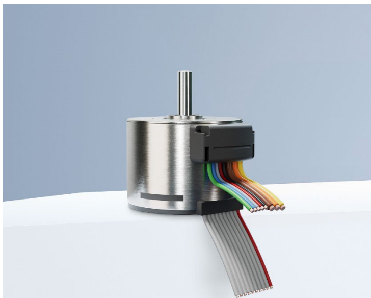
IERF3 L: il nuovo encoder incrementale di FAULHABER © FAULHABER
